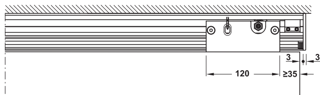
Schnitt Rollwagen 50 kg
