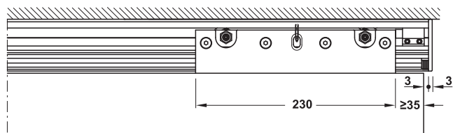
Schnitt Rollwagen 120 kg
