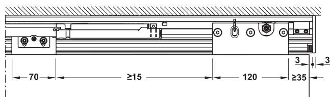
Schnitt Rollwagen 50 kg mit Dämpfung
